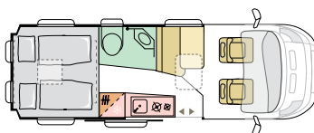
640 SGX | TWIN 60Y Elektrisches Hubbett
