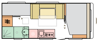
ALTEA 522 PK 60Y
