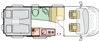
640 SGX PT | TWIN 60Y Pop TOP Dach und fixes Panoramafenster vorne
